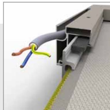
DETAIL ZIJGELEIDER + KABEL
